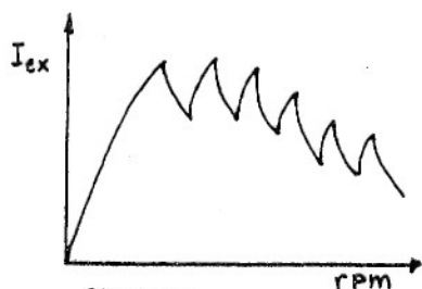
REGULADOR ELECTROMECAÁNICO
