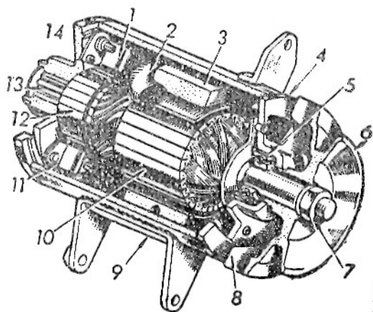
Dinamo cortada.
