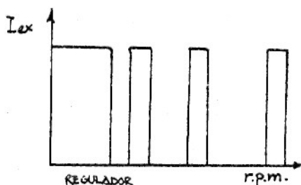
REGULADOR ELECTRONICO
