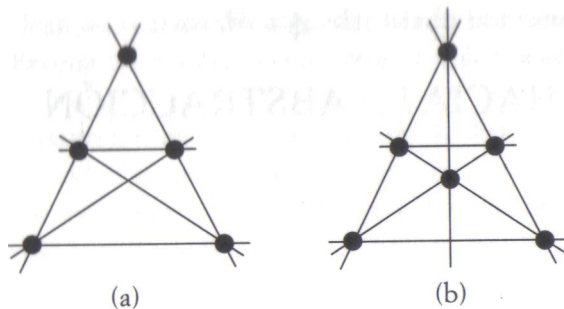
Figura 13: En estos diagramas cada punto está unido a todos los demás a través de líneas rectas. ¿Se puede construir un diagrama en el que cada recta contenga al menos tres puntos?
