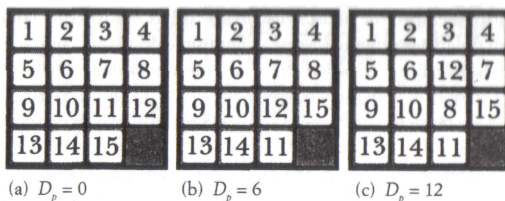
Figura 15: Desplazando las baldosas se consiguen varias disposiciones desordenadas. Se puede medir la cantidad de desorden en cada disposición a través del parámetro de desorden, D_p .
