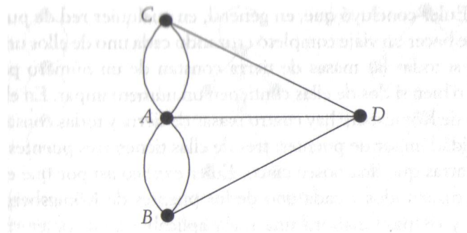
Figura 8: Representación simplificada de los puentes de Königsberg.
