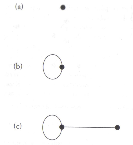
Figura 10: Euler probó su fórmula de redes demostrando que es válida para la red más simple y verificando a partir de ahí que continúa cumpliéndose sea cual sea la cantidad de añadidos que se sumen al vértice único original.
