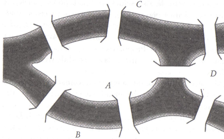
Figura 7: El río Pregel divide la ciudad de Königsberg en cuatro partes independientes, A, B, C y D. Siete puentes comunican las distintas partes y un acertijo local planteaba si era posible hacer una ruta de manera que cada puente se atravesara una única vez.
