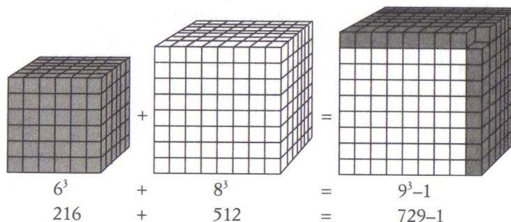
Figura 5: ¿Es posible unir los bloques de construcción de un cubo con los de otro para crear un tercer cubo aún mayor? En este caso, un cubo de 6 \times 6 \times 6 sumado a otro de 8 \times 8 \times 8 no reúne los bloques suficientes para formar un cubo de 9 \times 9 \times 9 . Hay 216 ( 6^3 ) bloques en el primer cubo y 512 ( 8^3 ) en el segundo. Entre los dos suman un total de 728 bloques que, a falta de uno, no bastan para alcanzar el valor de 9^3 .
