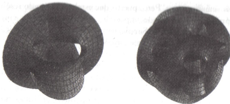
Figura 24: Estas superficies se crearon usando el programa de ordenador Mathematica. Son representaciones geométricas de la ecuación x^n + y^n = 1 , donde n = 3 para la primera imagen y n = 5 para la segunda. Aquí, x e y se consideran variables complejas.
