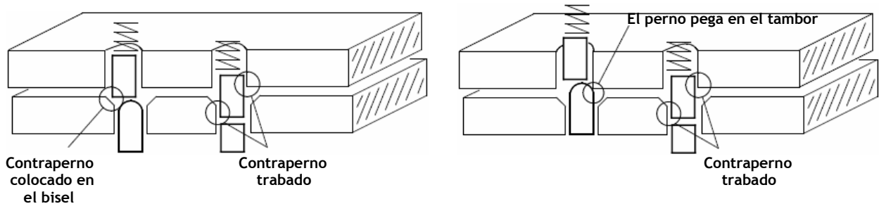
Figura 9.4: Perforaciones biseladas y pernos redondeados
