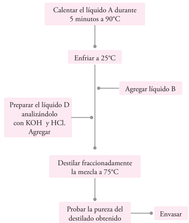
Figura 3.8 Diagrama de bloques.
