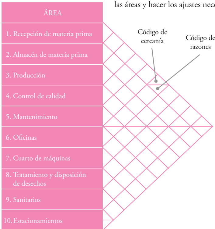
Figura 3.15 Diagrama de correlación de áreas.
