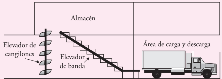
Figura 7.15 Transporte almacén-producción y almacén-carga y descarga.
