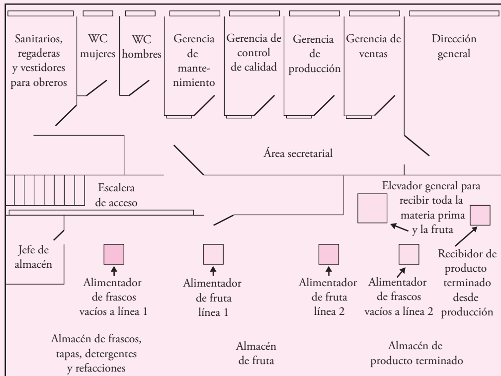
Figura 7.14 Alternativa 4. Nuevas áreas y nueva distribución de la planta alta.
