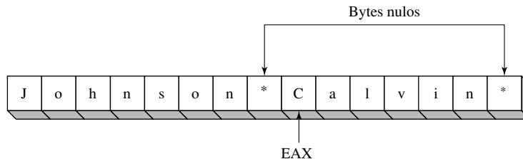
FIGURA 9-8 Ejemplo de Str_nextword .
