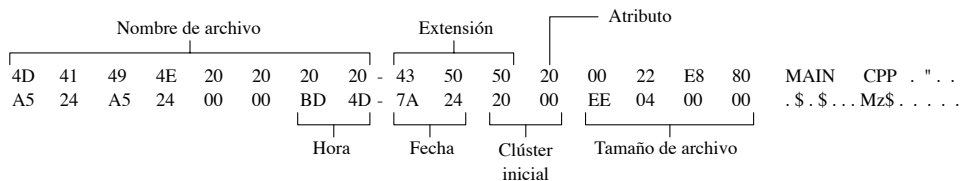
FIGURA 14-12 Ejemplo de entrada de directorio de un archivo.
