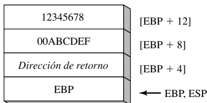
FIGURA 8-1 Marco de pila después de meter EBP.
