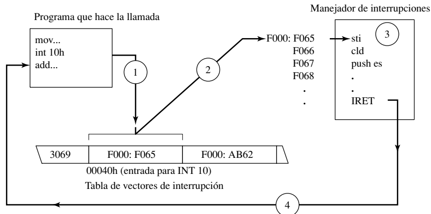
FIGURA 13-2 Proceso de vectorización de interrupciones.
