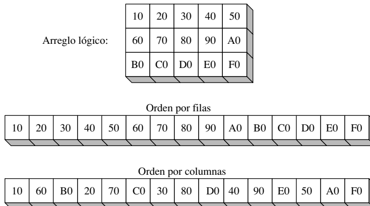
FIGURA 9-4 Orden por filas y por columnas.
