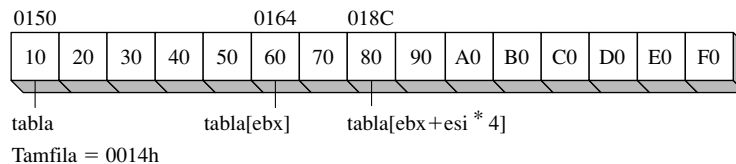
FIGURA 9-6 Ejemplo de base-índice-desplazamiento.
