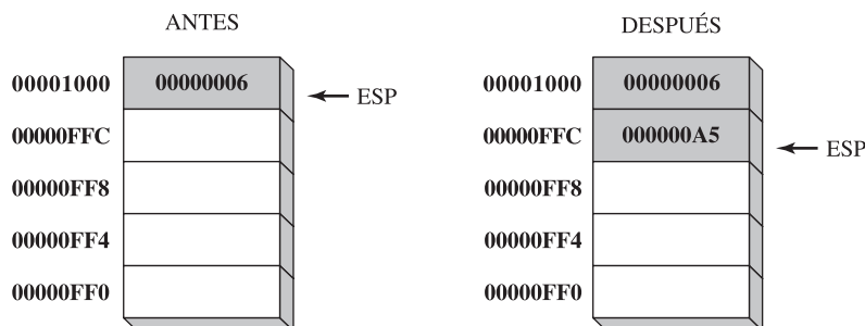
FIGURA 5-2 Meter enteros en la pila.
