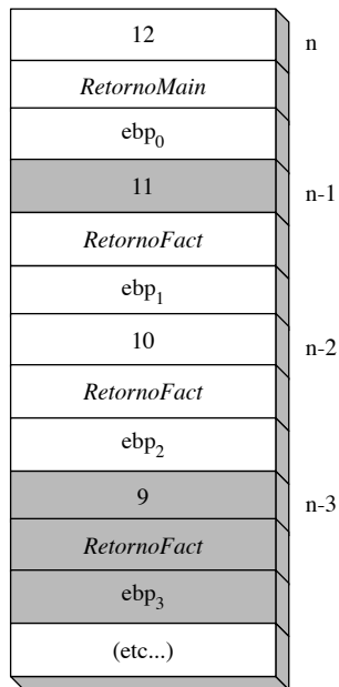
FIGURA 8-9 Marco de pila parcial, programa Factorial.
