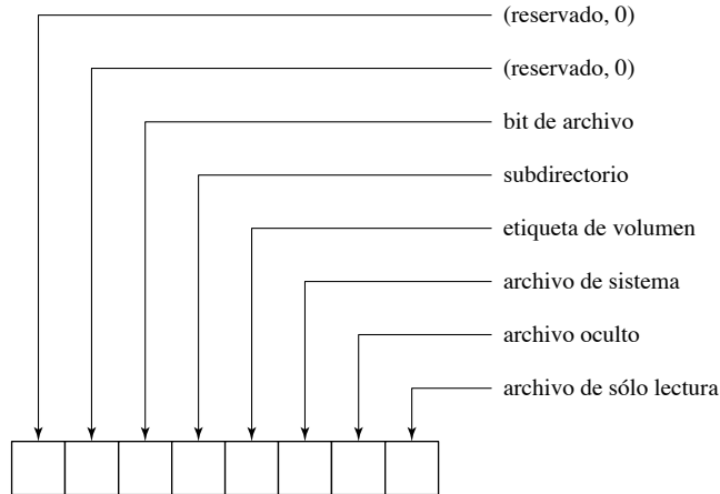
FIGURA 14-8 Campos de bytes de atributos de un archivo.
