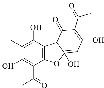
ácido úsnico
