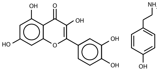
quercetina tiramina
