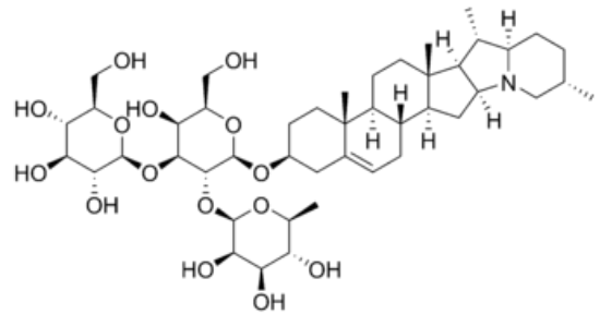
solanina
